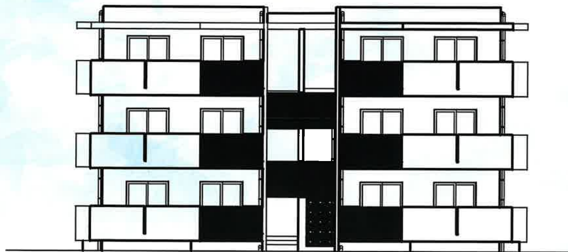
南側立面図
